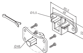
525.10061 макс. 30 Нм
