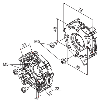
535.10093 макс. 30Нм
