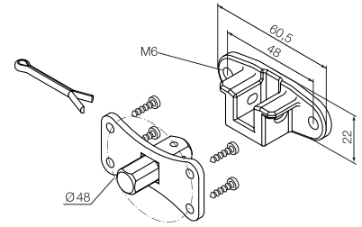
525.10056 макс. 30Нм
