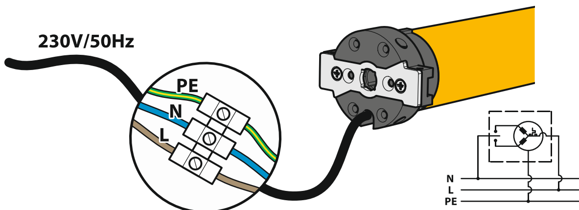
Bild 1. Elektrische Anschlüsse
